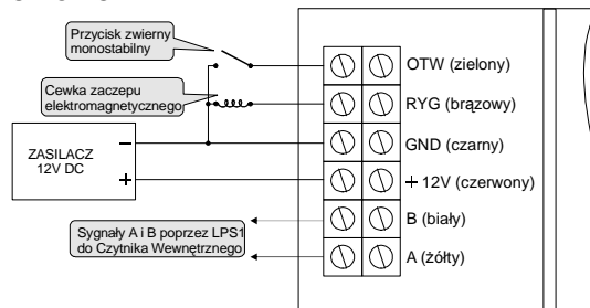
rys1. podłączenia czytnika RCP78R
