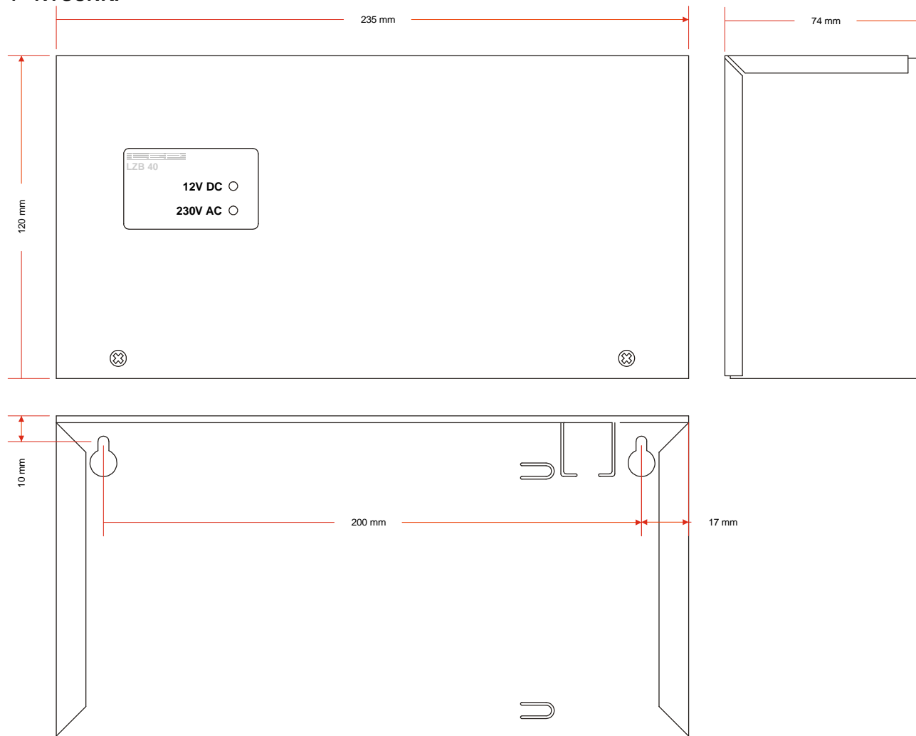
rys1. Zasilacz Buforowy LZB40 - wymiary główne
