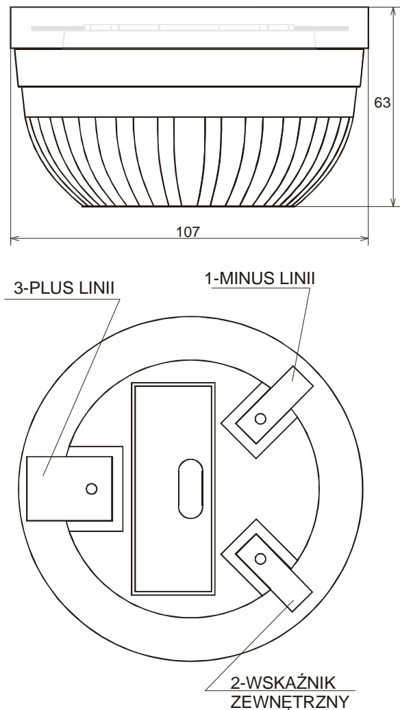
rys.2 Wymiary zewnętrzne czujki OSD23
