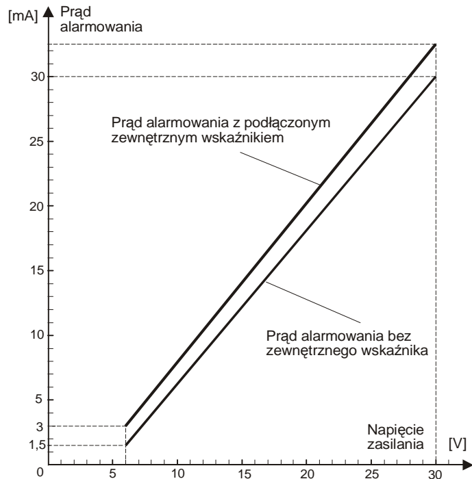
rys.1 Wykres prądu alarmowania czujki OSD23
